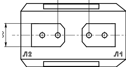
Рис. 5 - Общий вид трансформаторов тока ТОЛ-СВЭЛ-10-1 (2-8) на номинальные первичные токи 1200-2000 А. Остальное см. рис. 1
