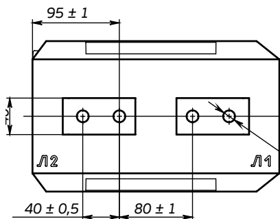
Рис. 1 - Общий вид трансформаторов тока ТОЛ-СВЭЛ-10-1
