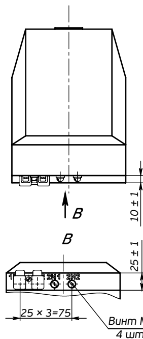
Рис. 3 - Общий вид трансформаторов тока ТОЛ-СВЭЛ-10-2. Остальное см. рис.1
