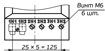
Рис. 2 - Общий вид трансформаторов тока ТОЛ-СВЭЛ-10-7. Остальное см. рис.1
